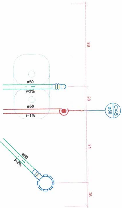
Detalhe S5 Escala 1:25
